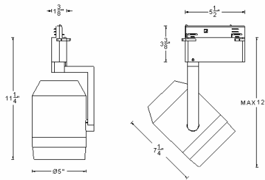
WHK-530-39E
