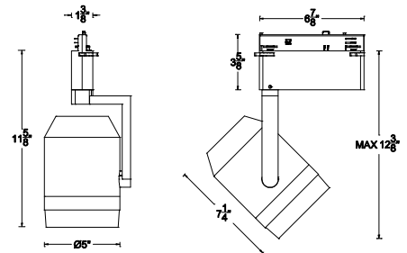
WTK-530-70E
