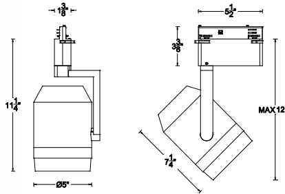
WTK-530-39E
