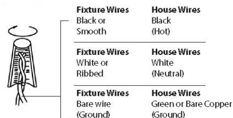
Fig. 2 Wiring
