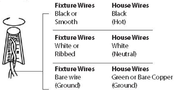
Fig. 2 Wiring
